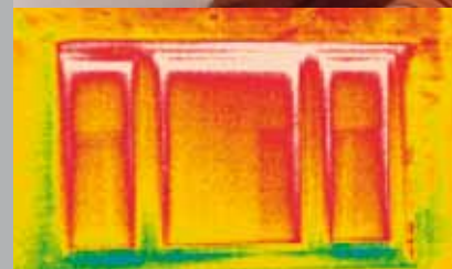
Voor de renovering: Rood geeft het gebied met warmteverlies aan.
